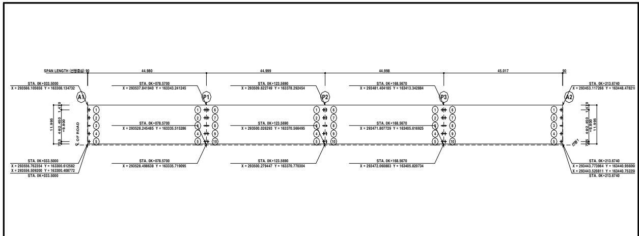
【그림 17.3.1】 교량반침 배치도
