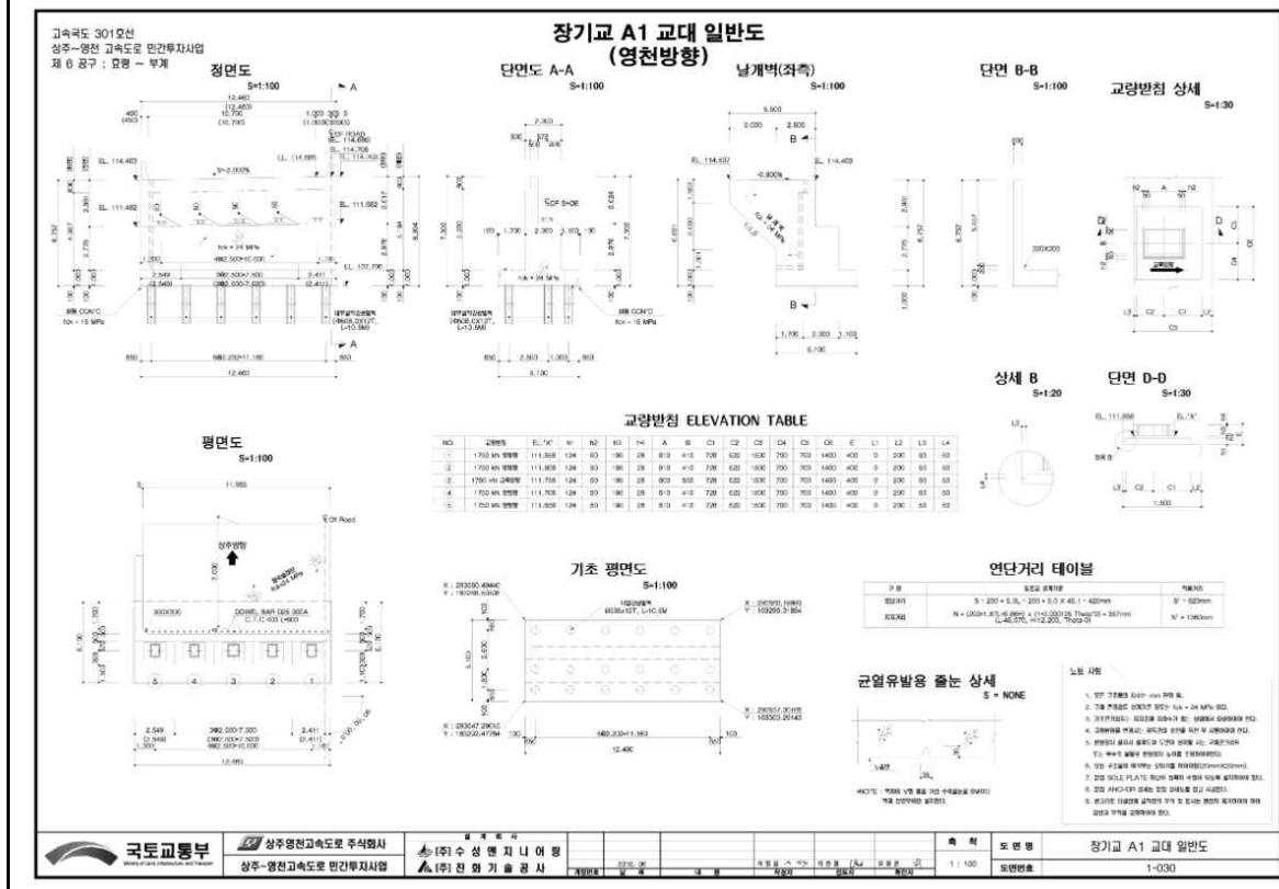
【그림 17.1.6】 교대 일반도
